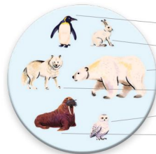
Ladovec
