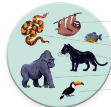
Džungľa
