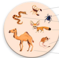
Púšť
